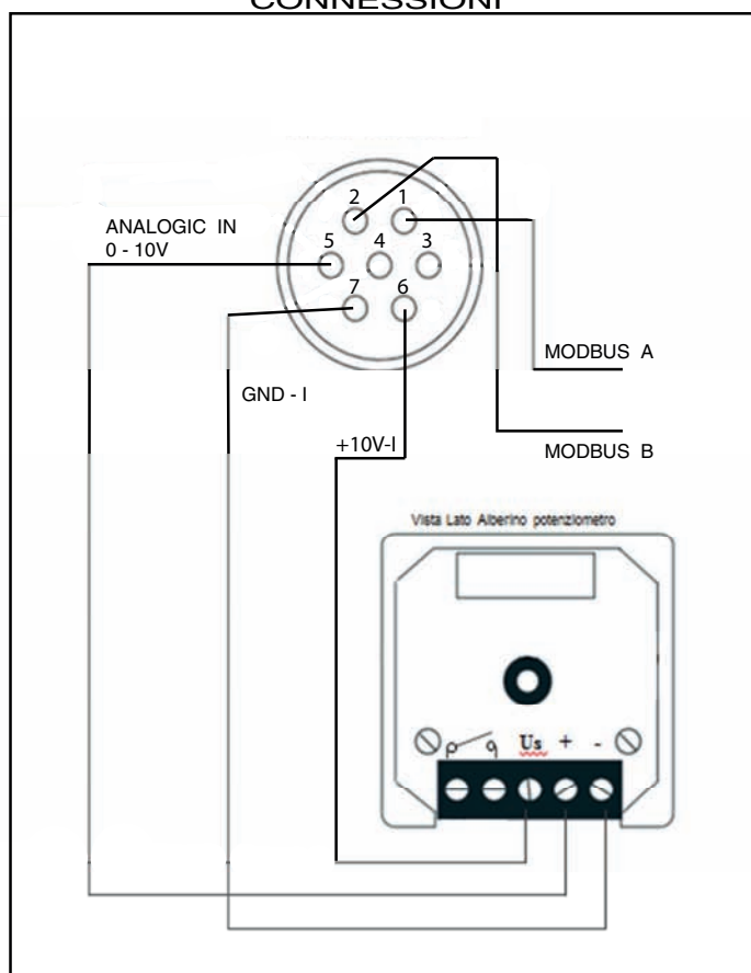
DETTAGLIO CONNESSIONI
